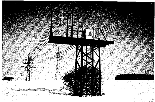
Figur 5 Testfreileitung
