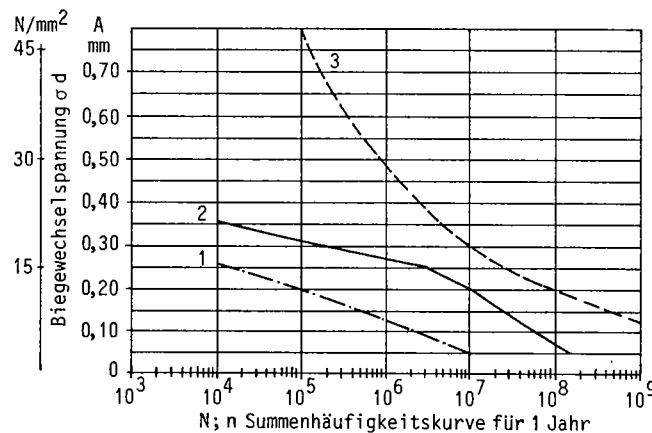
Figur 4 Typische Häufigkeitskollektive
